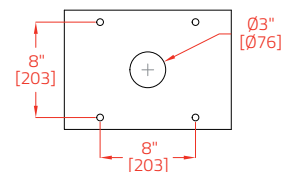
WXB-240 FOOTPRINT
