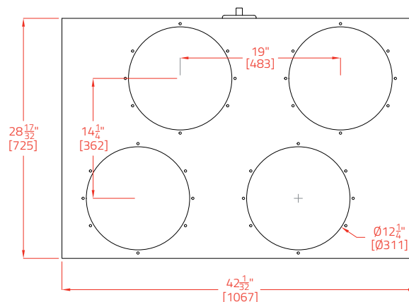
WXB-240 LID TOP VIEW
